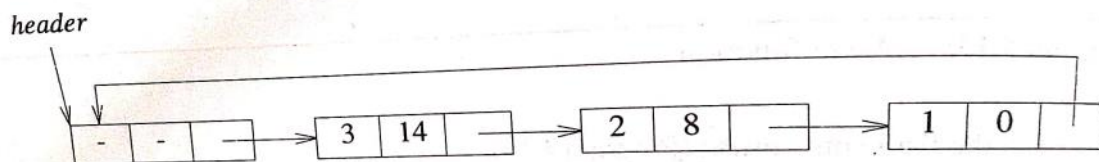
(b) 3x^{14} + 2x^8 + 1
